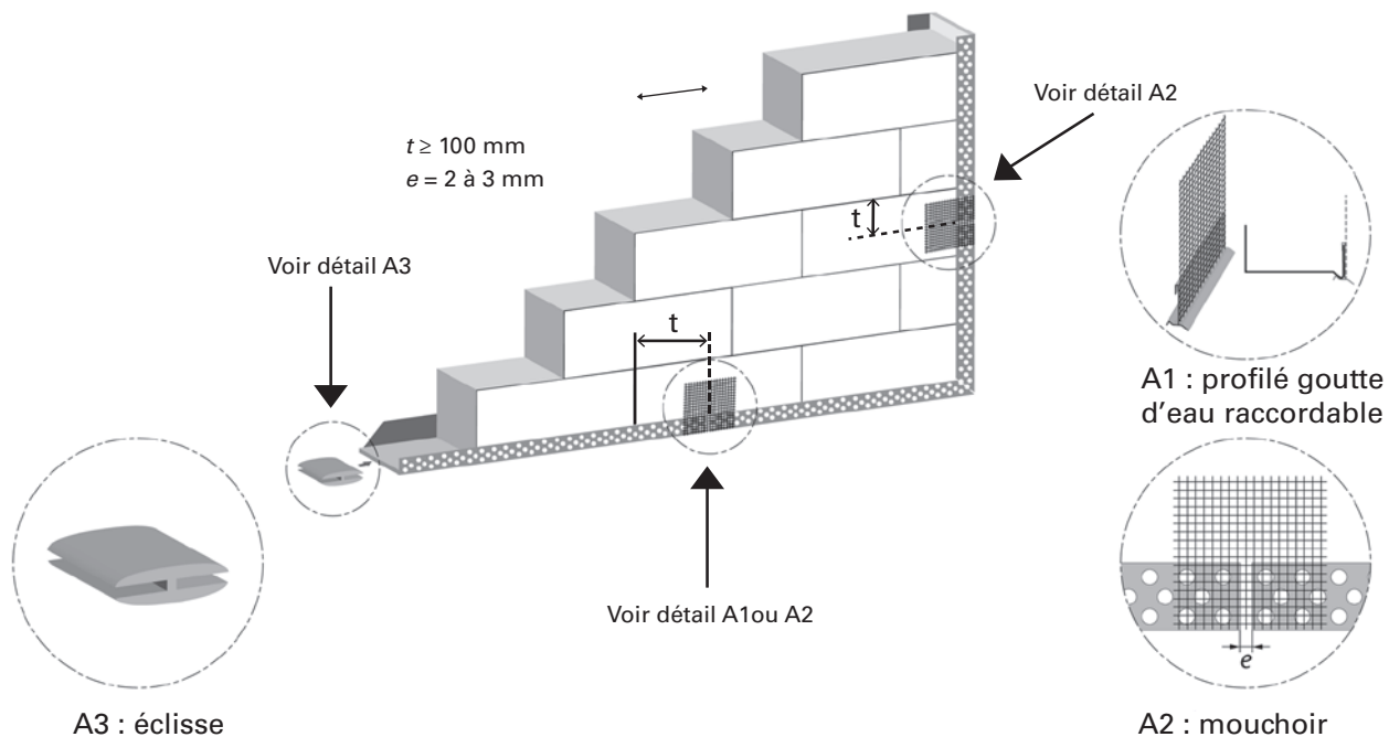
Figure 1 – Disposition des profilés de départ et latéraux – Renforts aux jonctions entre profilés
