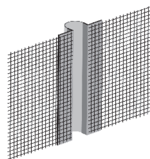
Profilé à soufflet
